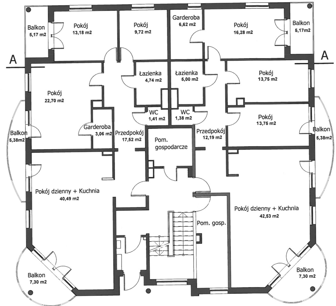
Lokal mieszkalny nr 2 Powierzchnia użytkowa: 111,50m 2
