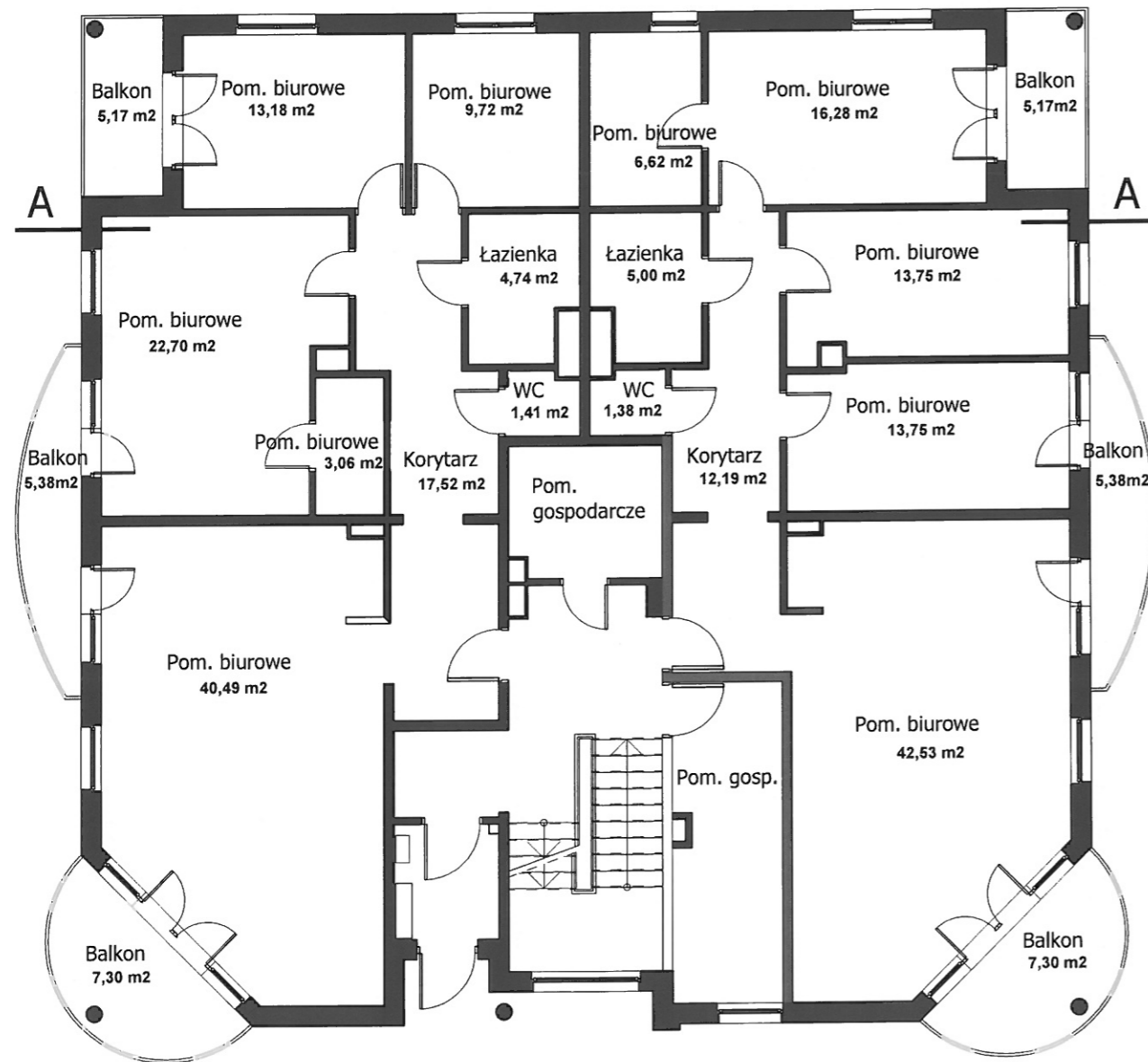
Lokal usługowy nr 2 Powierzchnia użytkowa: 111,50m 2
