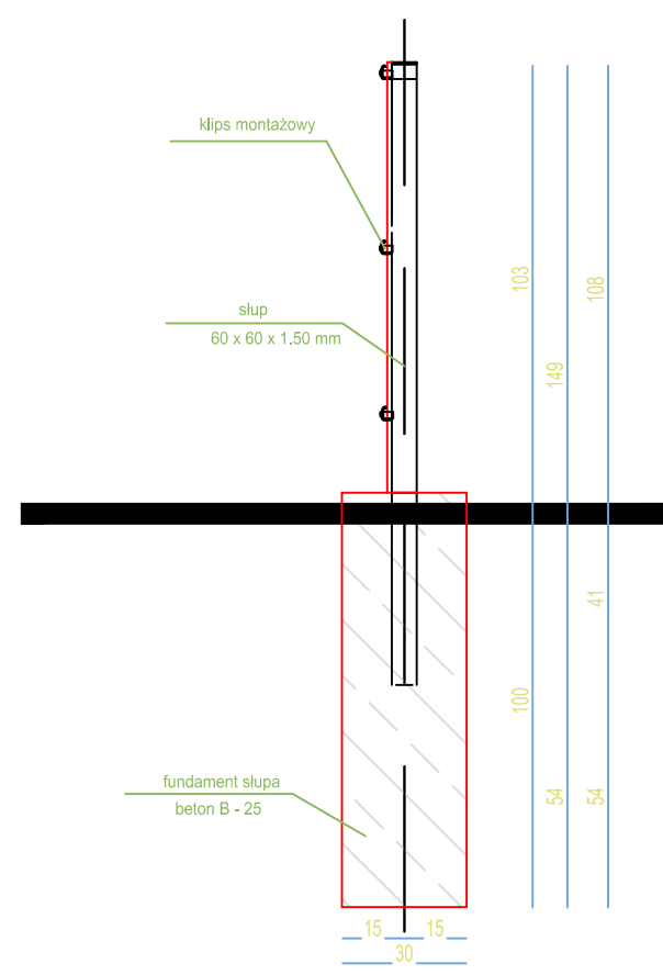
SEGMENT SYSTEMOWY OGRODZENIA - 250 CM PRZEKTÓJ
